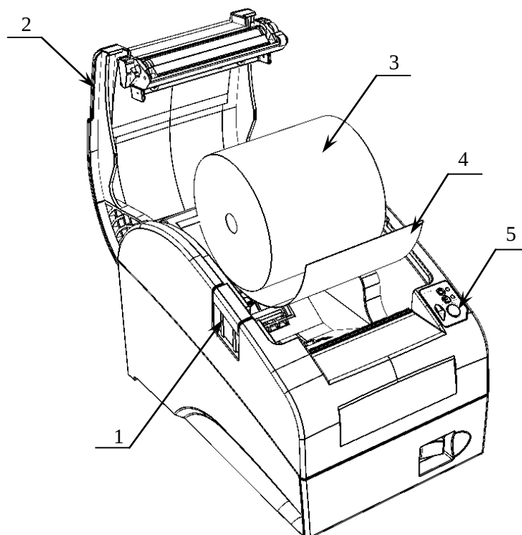
Рисунок 6. Заправка бумаги при горизонтальной установке ККТ
