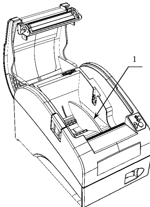
Рисунок 8. Установка ограничителя бумаги в ККТ.
